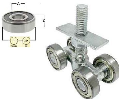
RODIZIO PARA PUERTA 4X1" METAL
