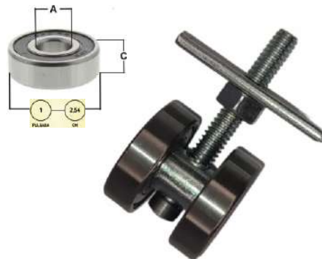
RODIZIO PARA PUERTA 2X1" METAL REF.
